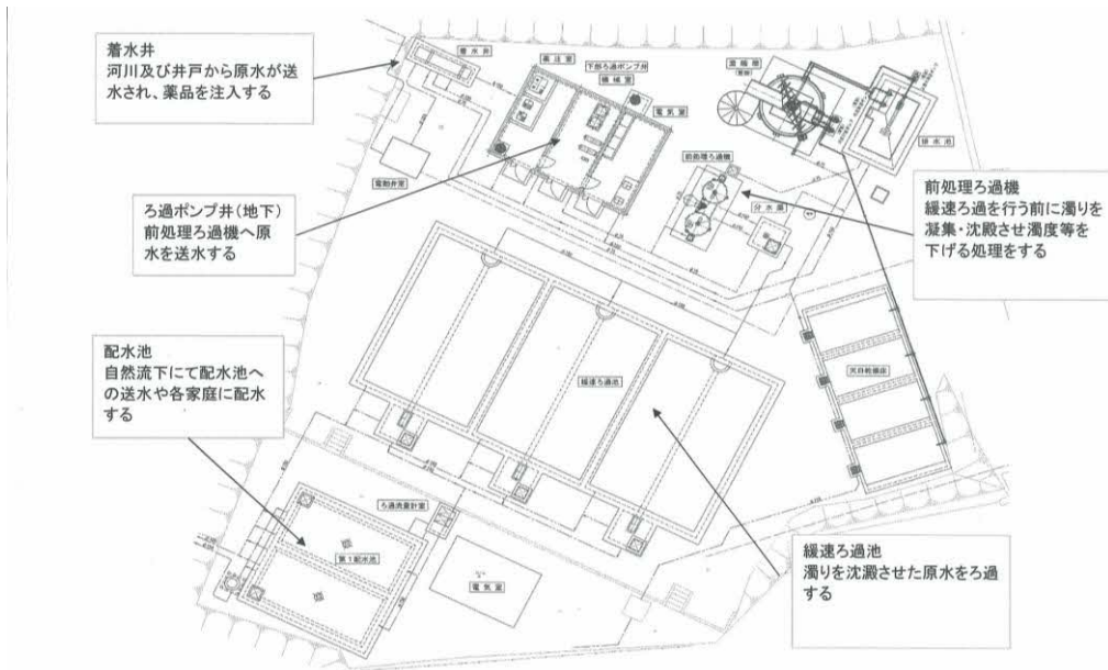
図-3 浄水フロー（緩速ろ過方式）
