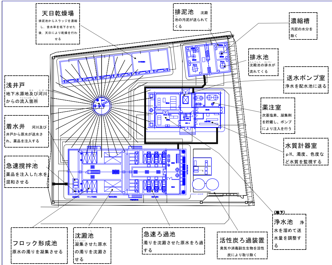
図-2 浄水フロー（急速ろ過方式）
