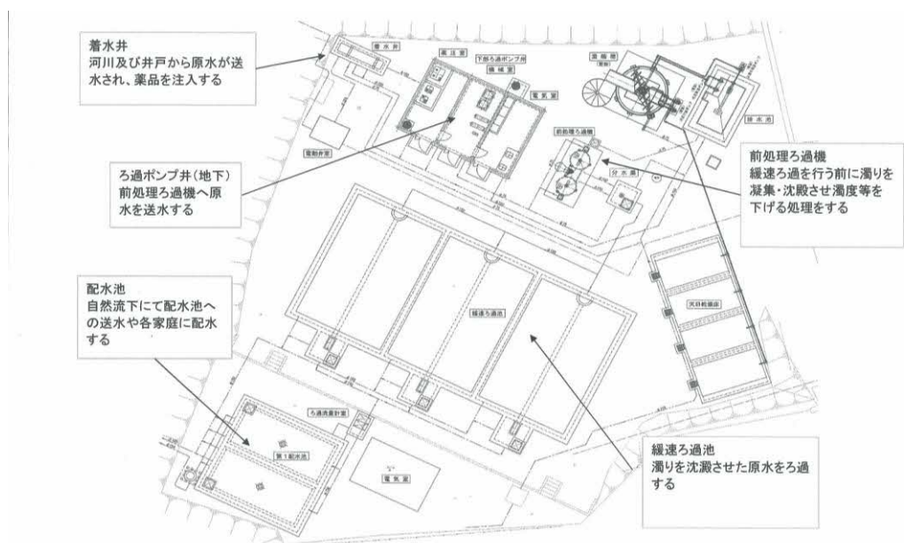
図－３ 浄水フロー（緩速ろ過方式）
