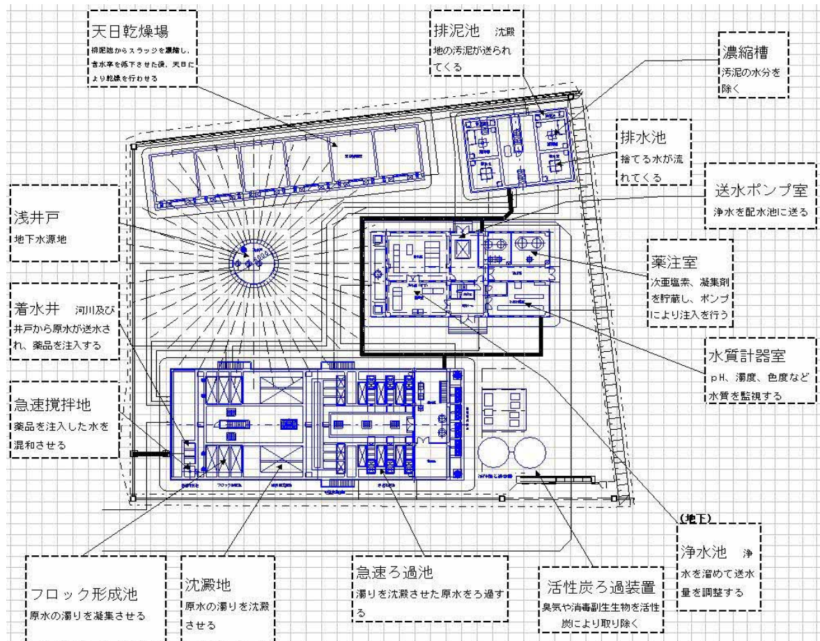
図－２ 浄水フロー（急速ろ過方式）
