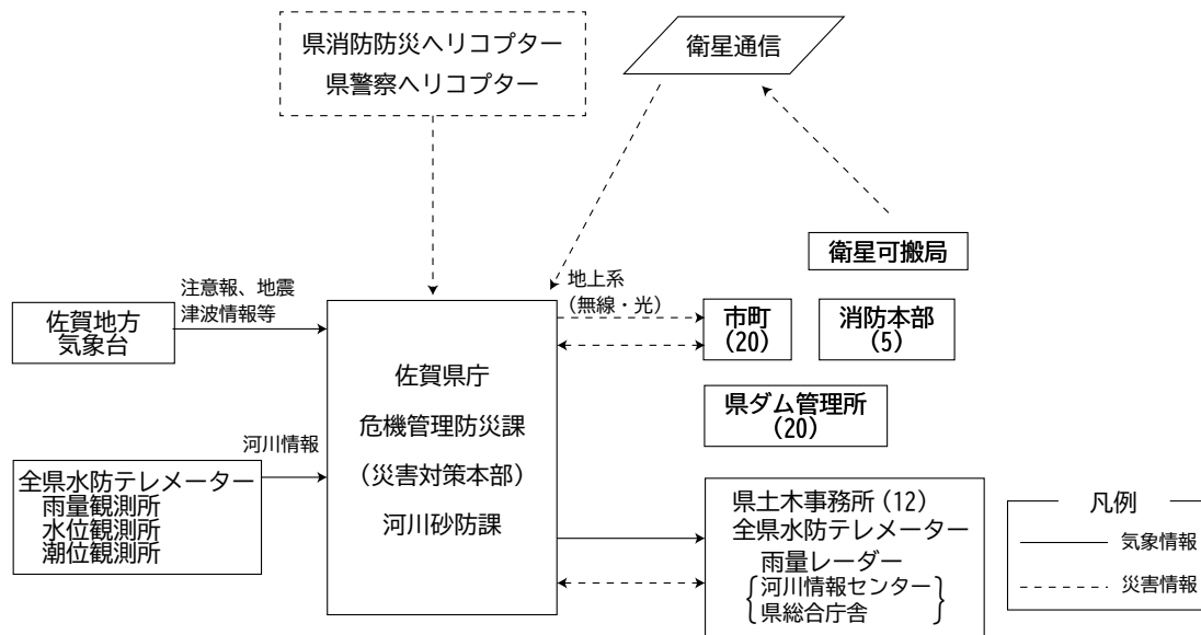
図 2-2 県防災情報システムの防災情報連絡系
