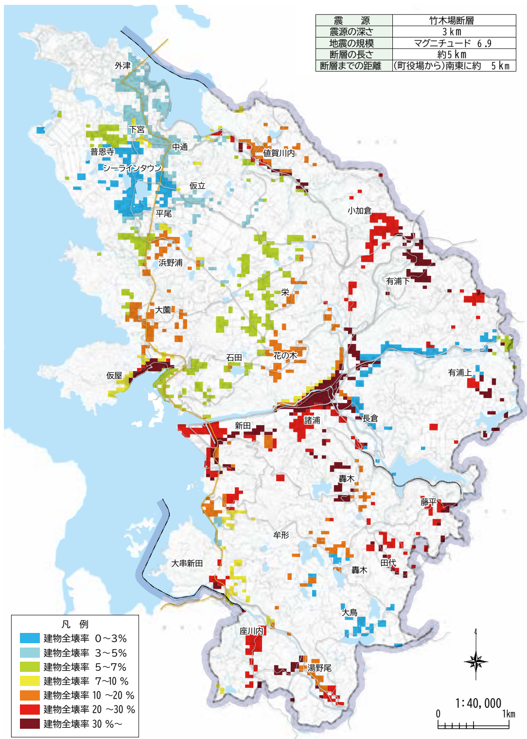
図 1-14 危険度マップ（建物の全壊率の分布）
