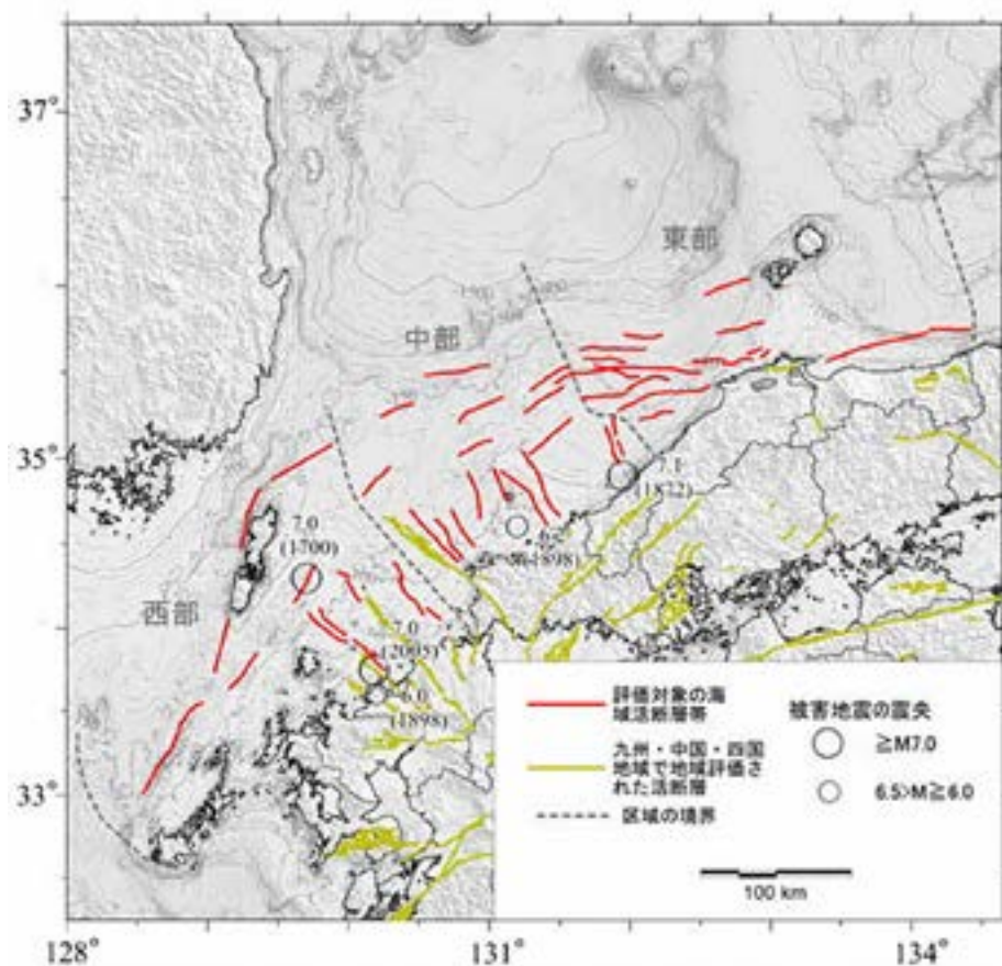
図 1-16 日本海南西部（評価対象海域）における評価対象の海域活断層と主な被害地震の震央 （出典：地震本部ホームページ）
